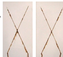
低温硬化型 従来型 【塩水噴霧試験 300時間(ペンタイト銅板)】
