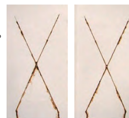
低温硬化型 従来型 【塩水噴霧試験 300時間(ベンタイト鋼板)】
